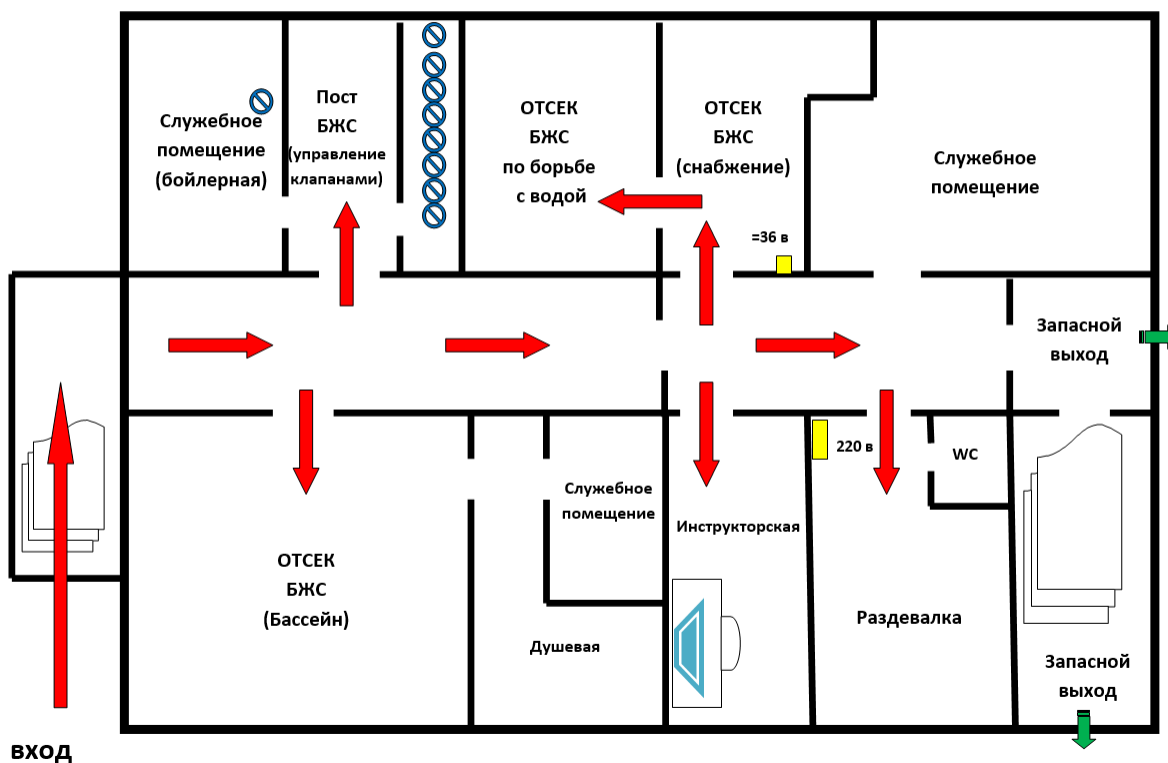
Схема тренажера по борьбе с водой
